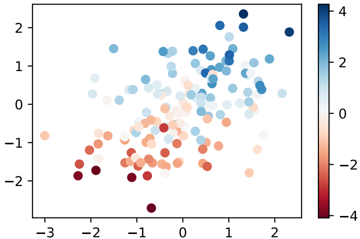
Linear
