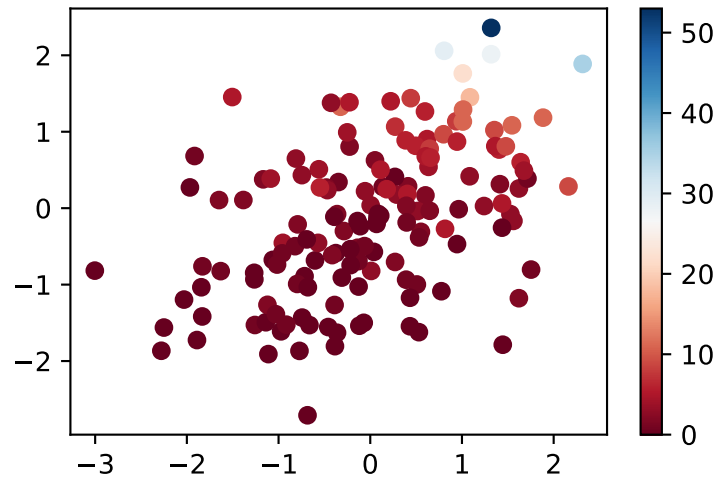
Poisson
